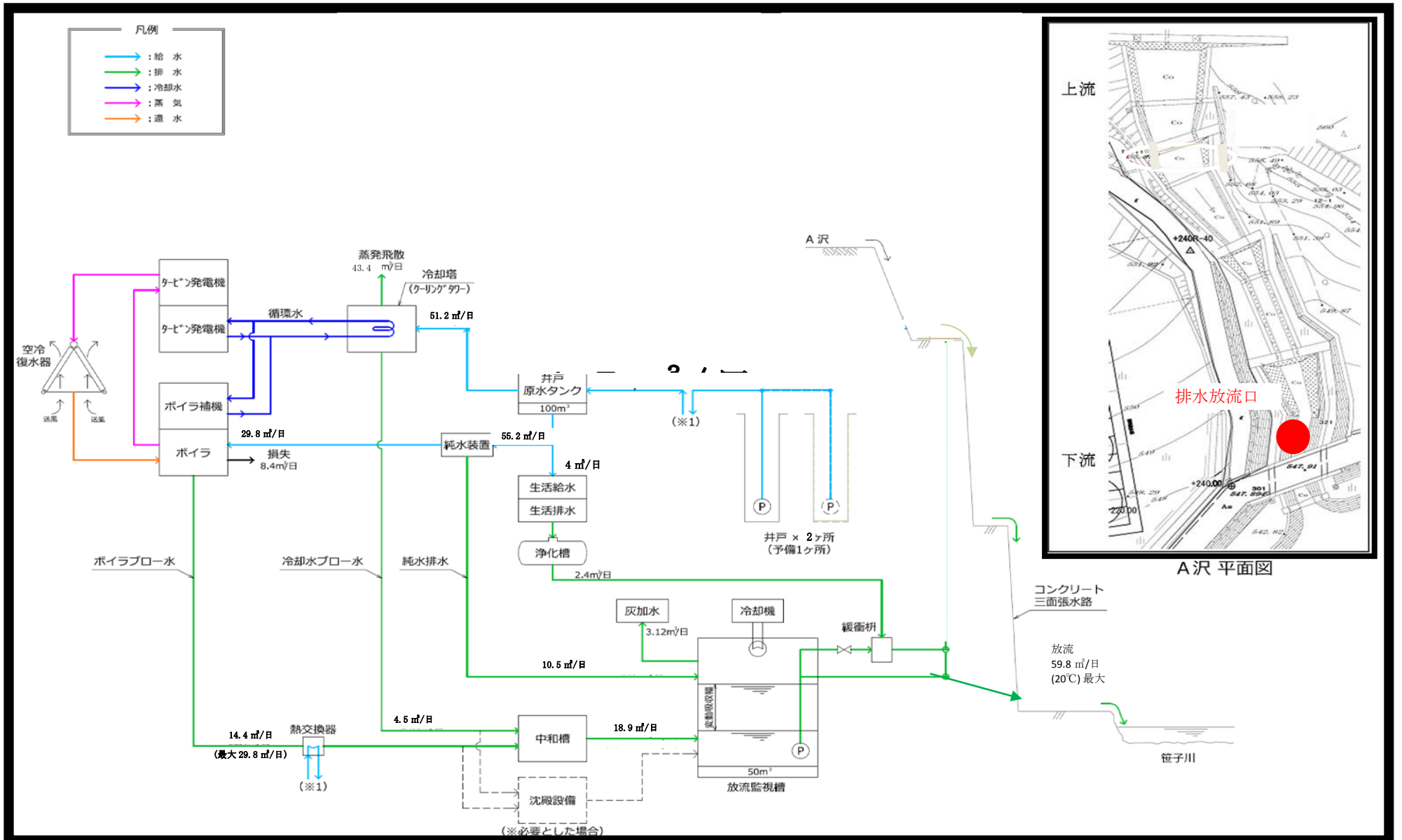
図 1-4-10 水収支フロー図
